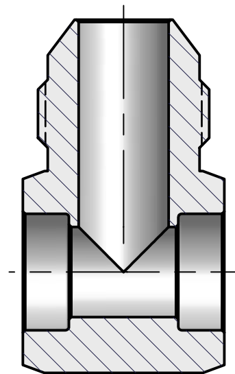
SECTION A-A SCALE 1.75 : 1
