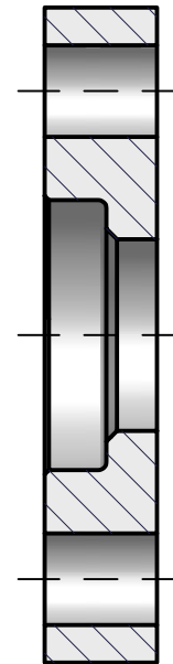
SECTION A-A SCALE 1 : 1
